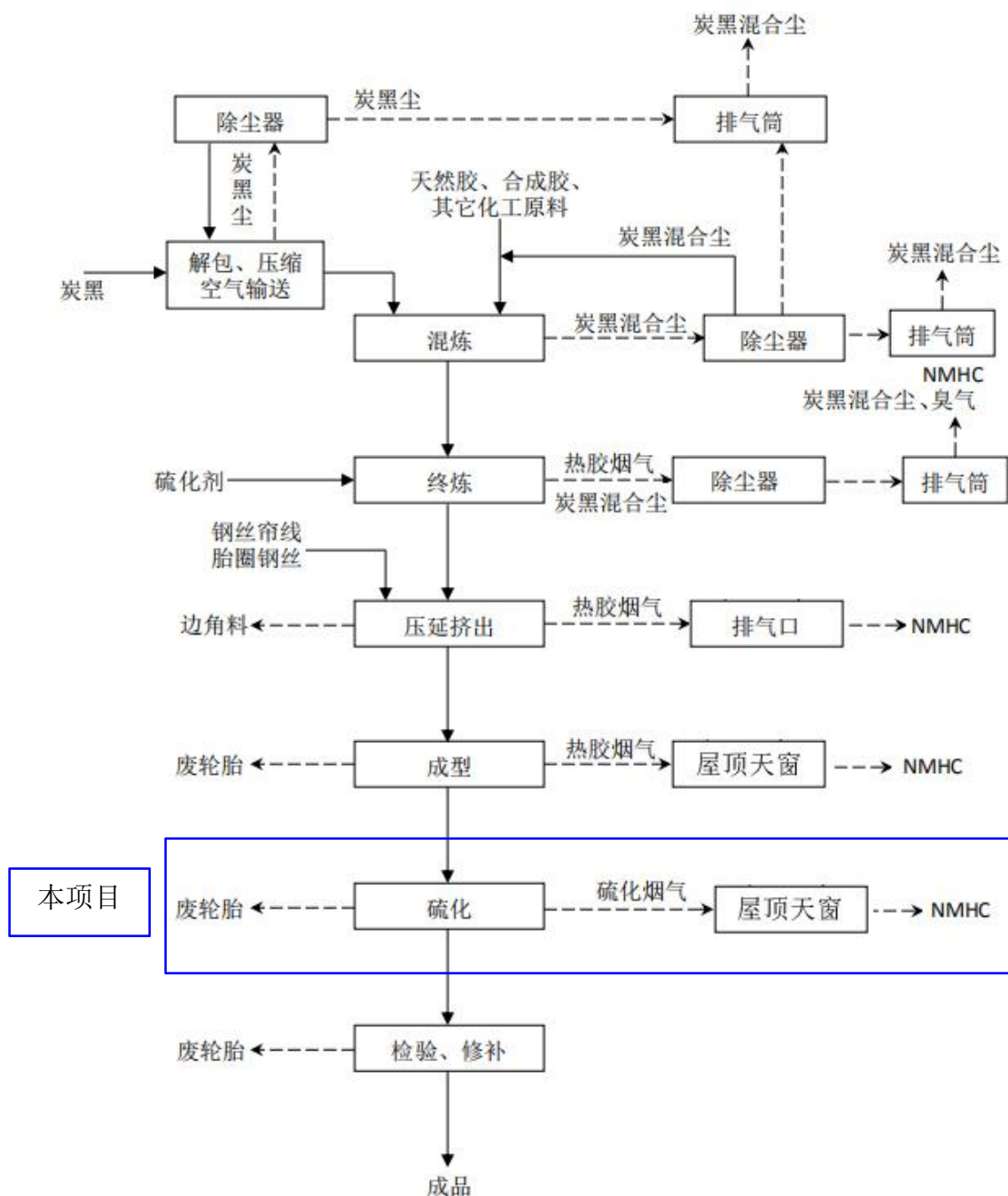
图 2.2-2 运营期硫化工段在轮胎生产过程中所处位置及产污节点图
